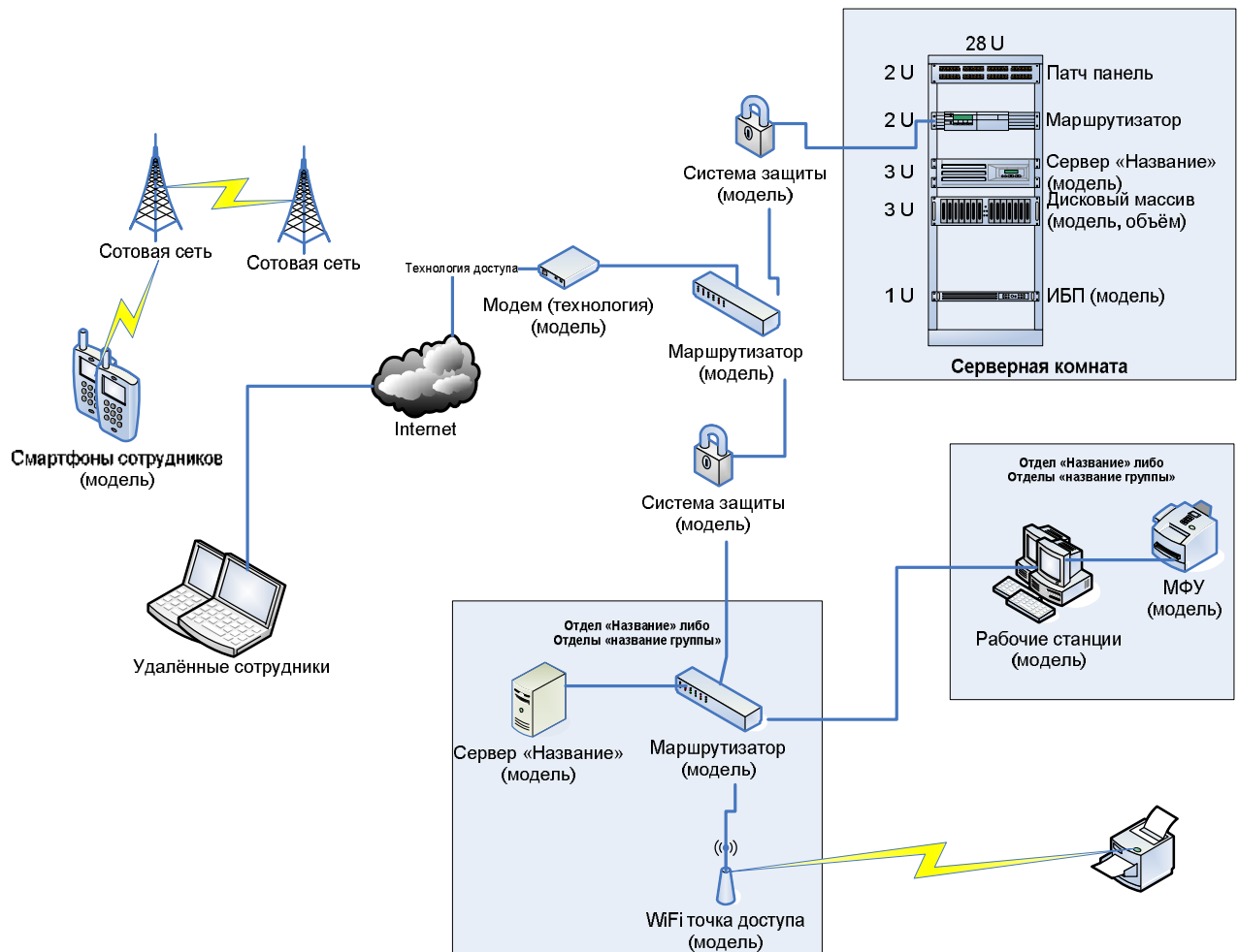
Общий пример представления технической архитектуры
