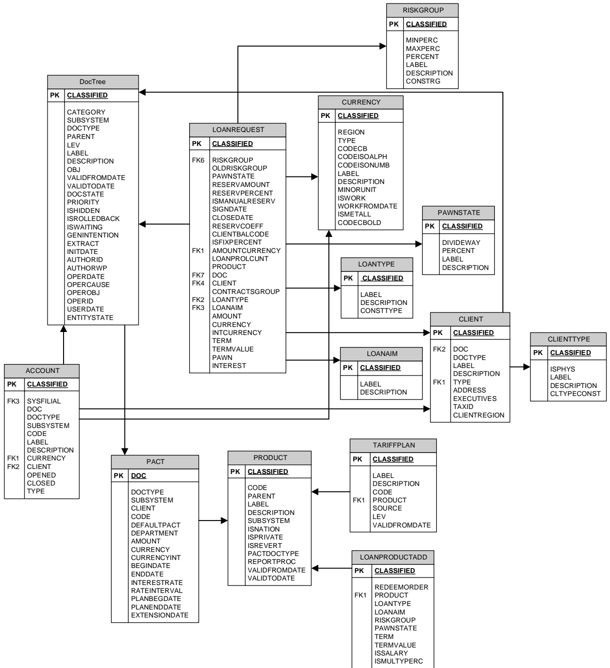
Пример фрагмента ER модели
